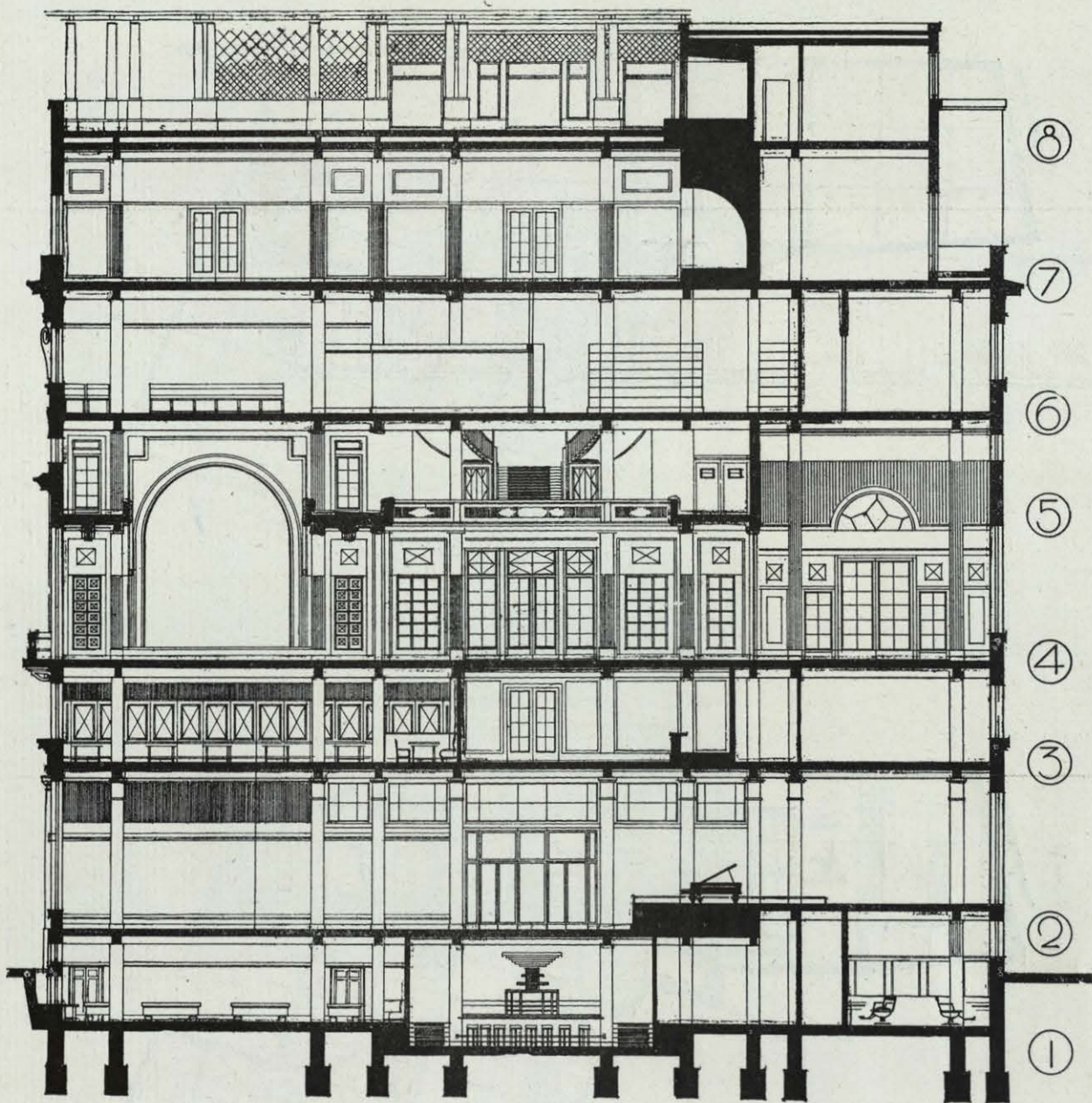
SECCIÓN.
