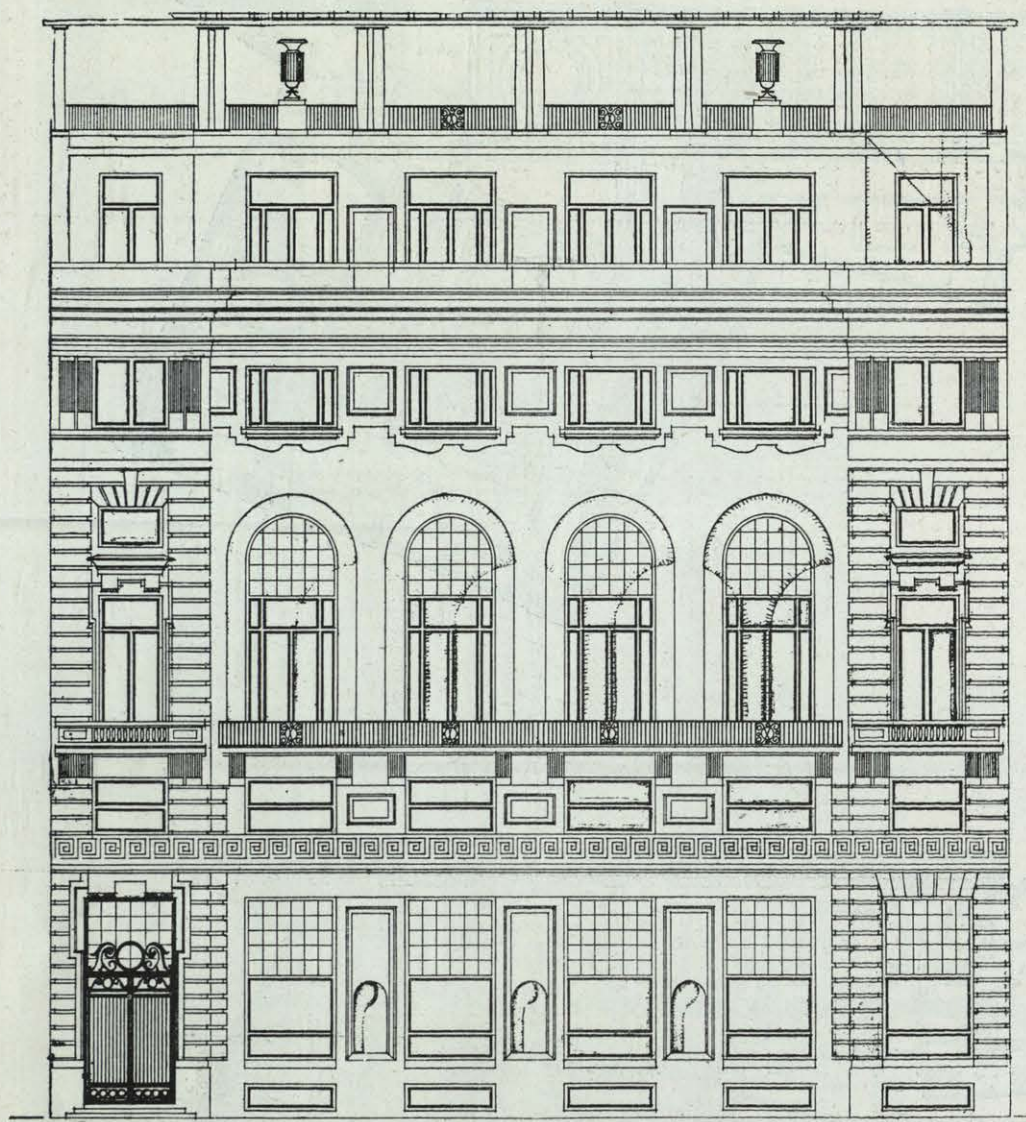
FACHADA PRINCIPAL.
